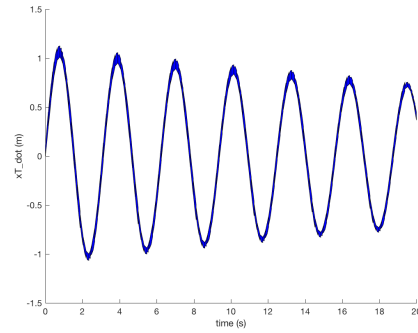
(b) Output - Displacement ( xT\_dot ).
